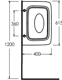
Pisuar Ara Bölme Urinal with Separator
