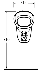
Üstten Su Girişli Pisuar Top Water Inlet Urinal
