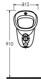
Arkadan Su Girişli Pisuar Back Water Inlet Urinal
