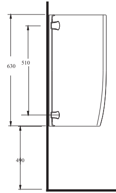
Pisuvar Ara Bölme Urinal with Separator
