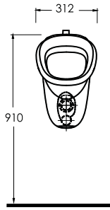
Üstten Su Girişli Pisuvar Top Water Inlet Urinal
