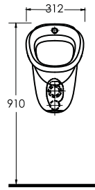
Arkadan Su Girişli Pisuvar Back Water Inlet Urinal
